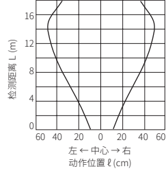
• BJR15M-TDT-F
