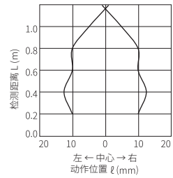
• BJR1M-DDT-F
