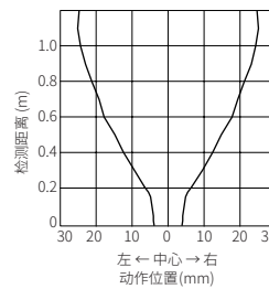
特性曲线 ③
