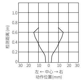
特性曲线 ④
