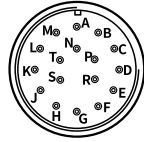
• 1-1/4-18UNEF-2A PIN 排列图
